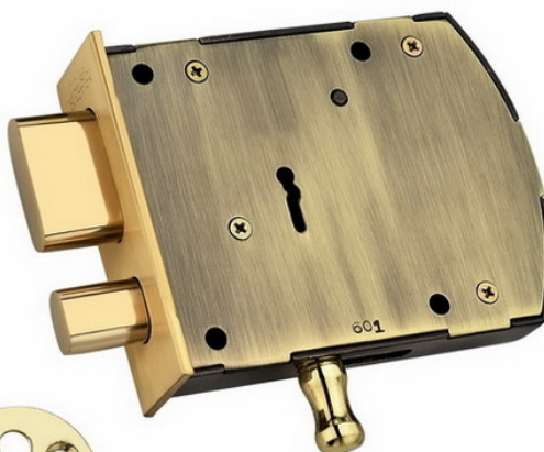
TULIP 8 LVS. SLEEK DOOR LOCK - ANTQ. 100 x 125 x 20mm KY
